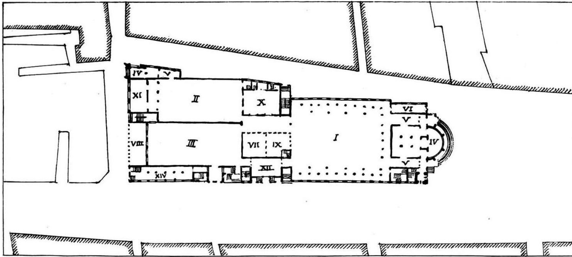
H.P. Berlage, Beurs, plattegrond, 1896
